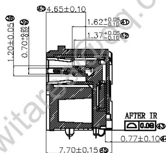
SECTION B-E
