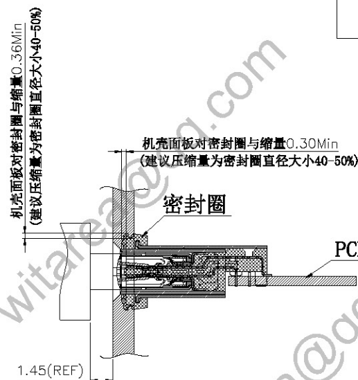
组装面板后公母头对插示意图
