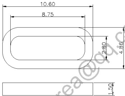
防水圈尺寸图
