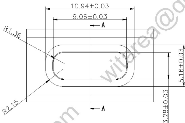
机壳开孔建议尺寸图
